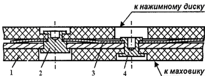
Рис. 116. Крепление накладок:
