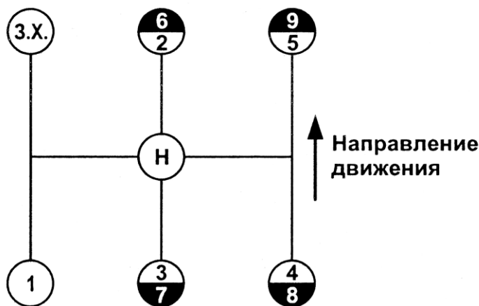
Рис. 96. Схема положений рычага переключения передач
