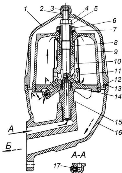
Рис. 17. Фильтр центробежной очистки масла:
