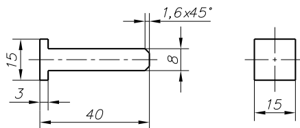
Рис. 105. Приспособление (материал – сталь)
