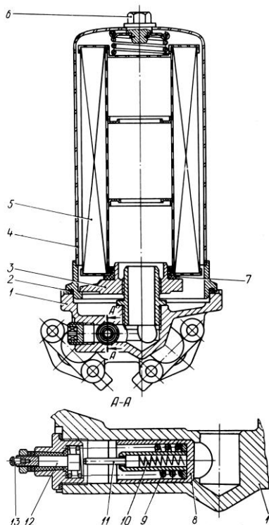
Рис. 16. Масляный фильтр:
