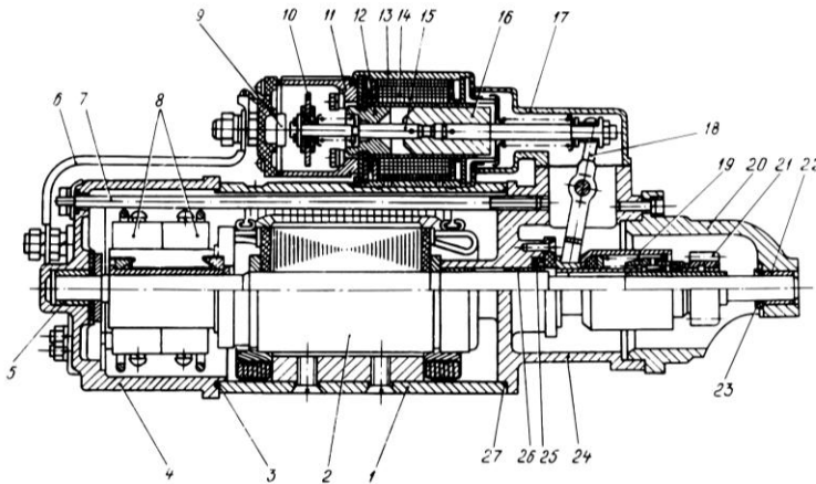
Рис. 40. Стартер:
