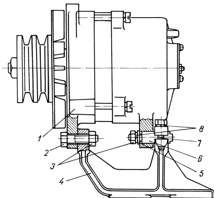
Рис. 70. Крепление генератора на двигателе:
