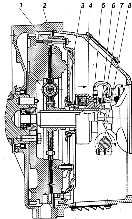
Рис. 91. Сцепление:
